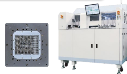
利用Socket確保封裝後的晶片功能特性及良率
